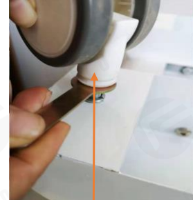
5. rögzítse a 4 kereket
